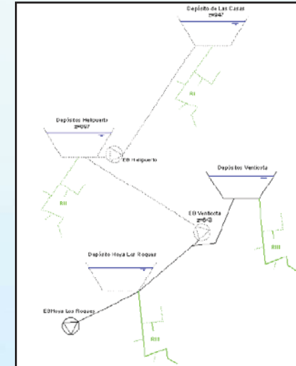
Funcionamiento hidráulico de las impulsiones de agua desalada
